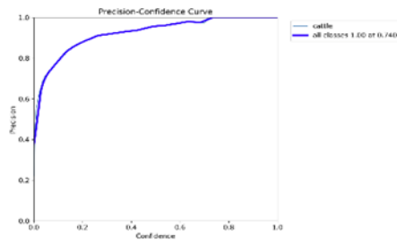
Fig. 11 - Precision-Confidence
